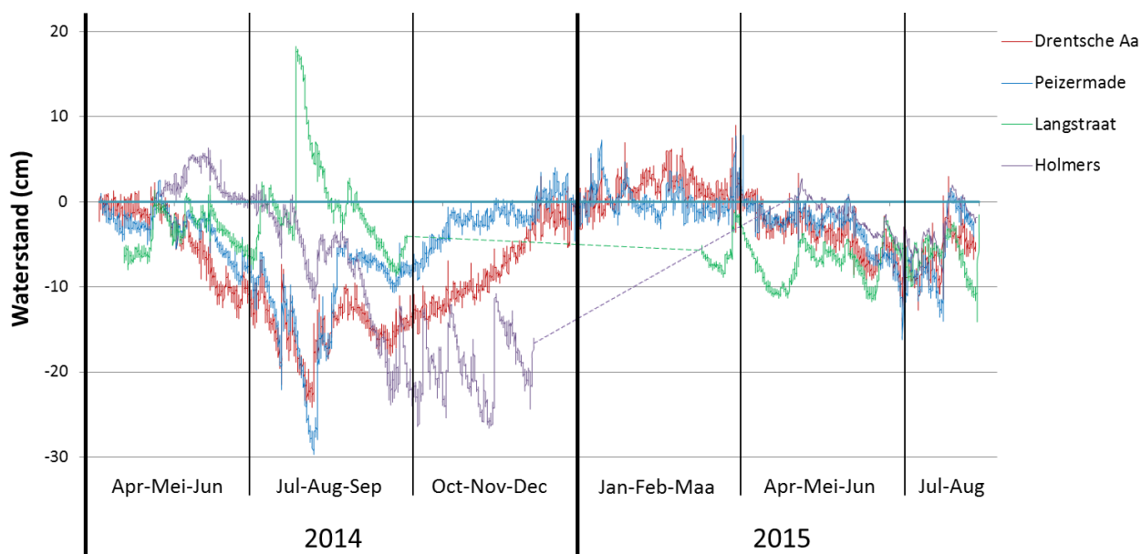
Figuur 67: Waterstanden in de vier studiegebieden gedurende de studieperiode. Ontbrekende data (gebieden HO en LS) zijn aangegeven met stippellijn.
