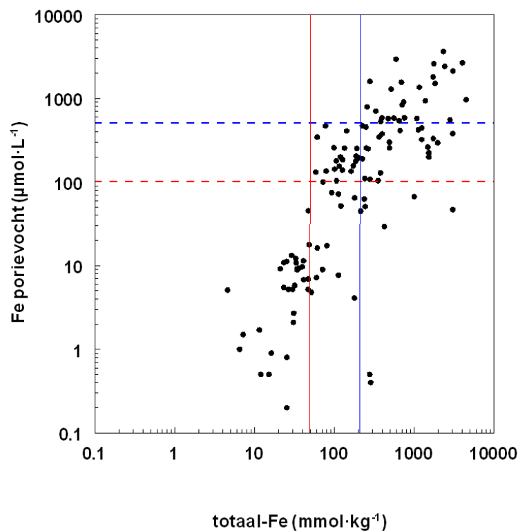
Figuur 11: IJzer in het porievocht in relatie tot ijzergehalten van de bodem. De blauwe lijn geeft de grens van ijzer in de bodem weer waarbij ijzertoxiciteit zeer waarschijnlijk een grote rol zal spelen bij vernatting. De rode lijn geeft de grens waarde waarboven ijzergehalte in de bodem waarbij ijzertoxiciteit differentiërend kan zijn voor de vegetatie.
