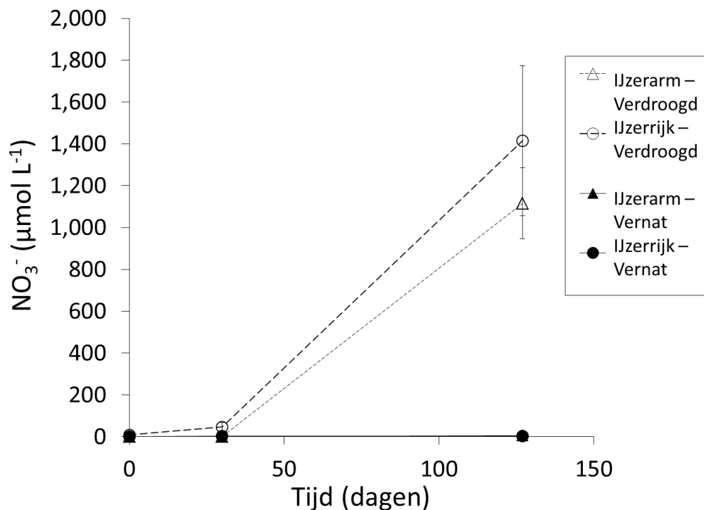
Figuur 61: Mobilisatie van nitraat ( \text{NO}_3^- ) met de tijd ( t = 0, 30 en 127 dagen) in het porievocht van 40 veenkolommen (gemiddelden van alle dieptes). Kolommen werden geclusterd in 4 groepen (telkens met 10 kolommen verspreid over 2 sites): vernatte-ijzerarme kolommen, verdroogde-ijzerarme kolommen, vernatte-ijzerrijke kolommen en verdroogde-ijzerrijke kolommen. De punten geven groeps gemiddelden weer \pm standaardfout.
