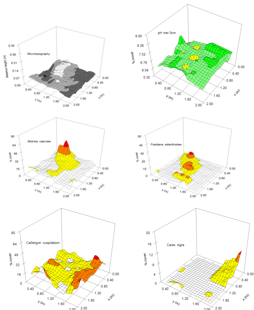
Hoogteverdeling, bodem pH en de bedekking van enkele planten en mossorten per 25*25 gridcel (Cirkel et al. 2012; Van der Ploeg et al. 2012.).
