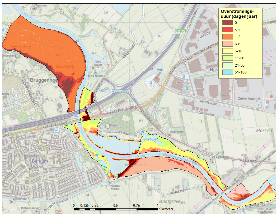
FIGUUR 2.7 OVERSTROMINGSDUUR IN MEEST BOVENSTROOMSE DEEL VECHT, BOVEN ZONDER REKENING TE HOUDEN MET DREMPELS, ONDER REKENING HOUDEND MET DREMPELS IN DE VORM VAN OEVERWALLEN EN KADEN.
