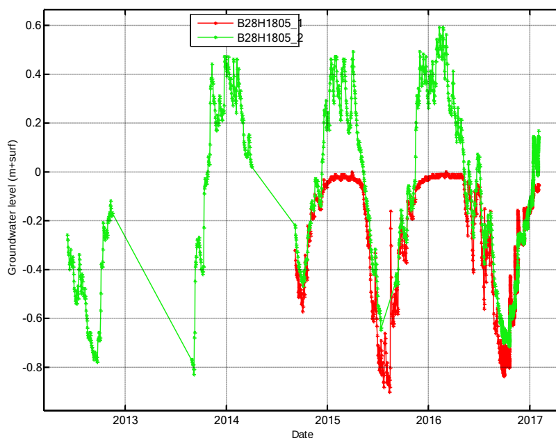
Figuur 10: Tijd-stijhoogtegrafiek van peilbuis B28H1805 (zelfde locatie als 1882, maar ondiepere filters op 1,2 en 4,5 m onder maaiveld).
