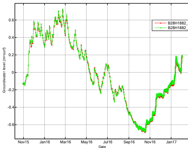
Figuur 9: Tijd-stijhoogtegrafiek van peilbuis B28H1882.
