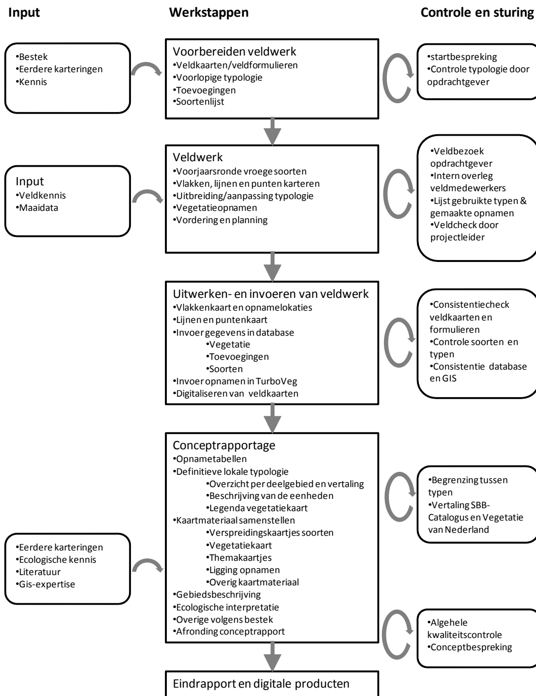
Figuur 3.1 - Methode (werkstappen, controle en sturing) vegetatiekartering
